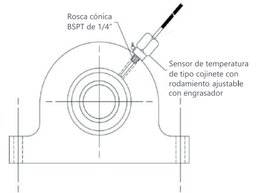
Esquema de instalación del sensor.
